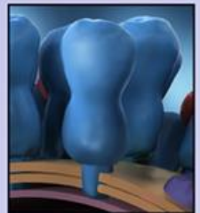
Hemagglutinin
